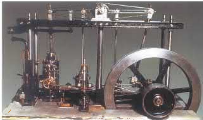
Первая универсальная паровая машина Джеймса Уатта построенная в 1784 году
