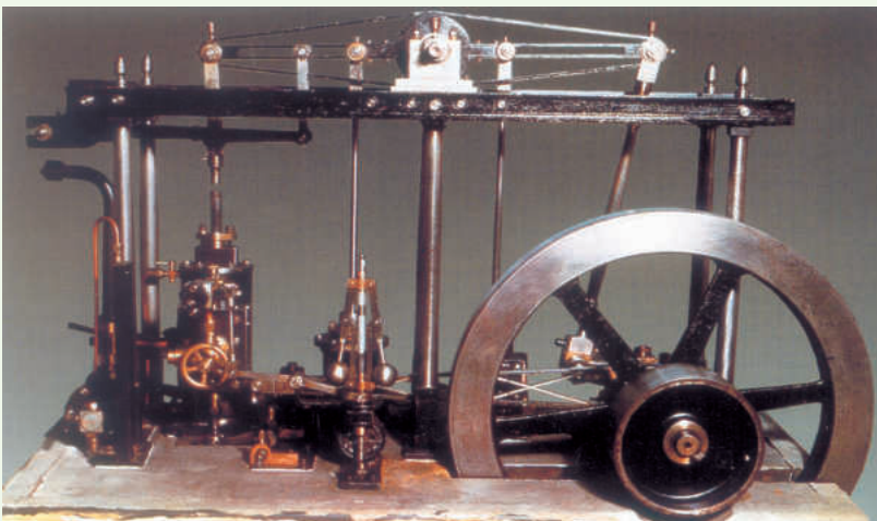
Первая универсальная паровая машина Д. Уатта
