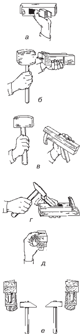
Рис. 1.17. Наладка ножа рубанка: а — удержание рубанка левой рукой; б — разборка ножа рубанка; в — установка ножа рубанка; г — окончательное закрепление лезвия; д — проверка правильности установки ножа; е — правка ножа рубанка
