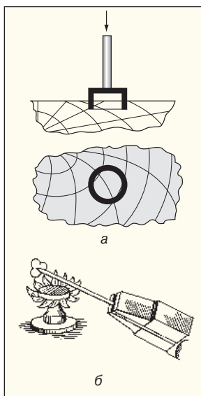
Рис. 1.36. Выжигание штамповкой: а — круглым штампом; б — нагревание штампов на горелке газовой плиты
