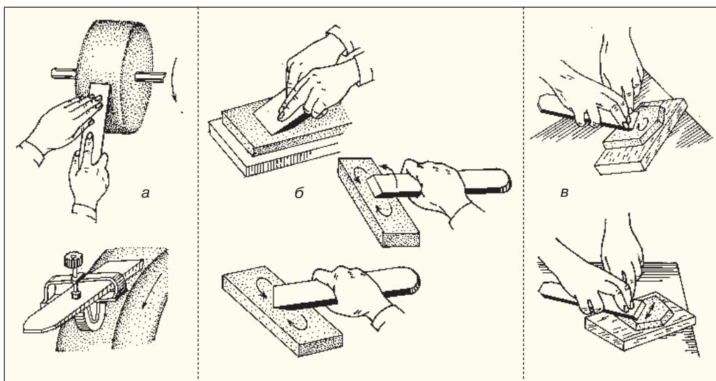
Рис. 1.13. Заточка ножей рубанка:
