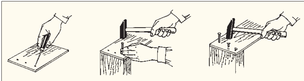
Рис. 1.29. Соединение гвоздями
