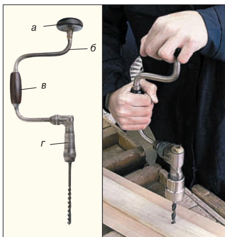
Рис. 1.25. Коловорот и операция сверления отверстия: а — деревянный грибок, б — скоба (стальное колено), в — ручка, г — патрон; операция сверления
