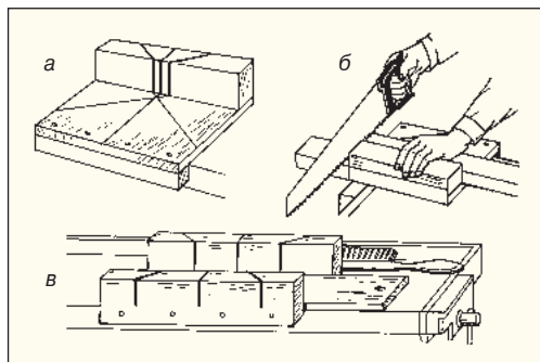
Рис. 1.23. Методы, облегчающие пиление доски:
