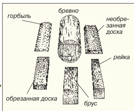
Рис. 1.3. Виды пиломатериалов
