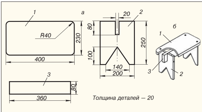
Рис. 1.15. Чертежи деталей (а) и технический рисунок (б)
