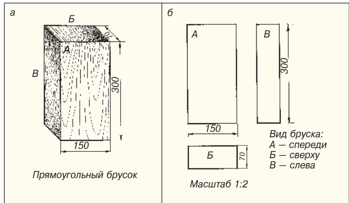
Рис. 1.12. Технический рисунок (а) и чертёж бруска (б)
